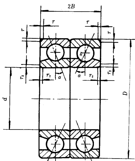
图 7 锁口在内圈上的成对双联 角接触球轴承(背靠背)
