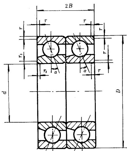
图 9 锁口在内圈上的成对双联 角接触球轴承(串联)
