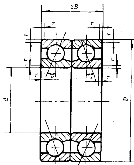
图 8 锁口在内圈上的成对双联 角接触球轴承(面对面)
