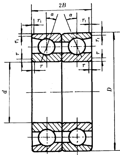
图 3 成对双联角接触球轴承 (背靠背) 70000 C/DB 型( \alpha=15^\circ ) 70000 AC/DB 型( \alpha=25^\circ ) 70000 B/DB 型( \alpha=40^\circ )
