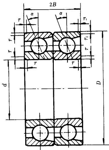
图 3 成对双联角接触球轴承 (背靠背) 70000 C/DB 型( \alpha=15^\circ ) 70000 AC/DB 型( \alpha=25^\circ ) 70000 B/DB 型( \alpha=40^\circ )
